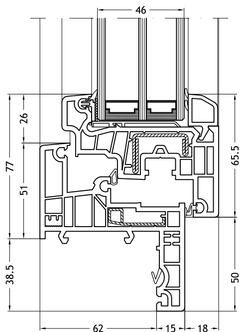
Telaio a Z 965 con anta Slim-line
