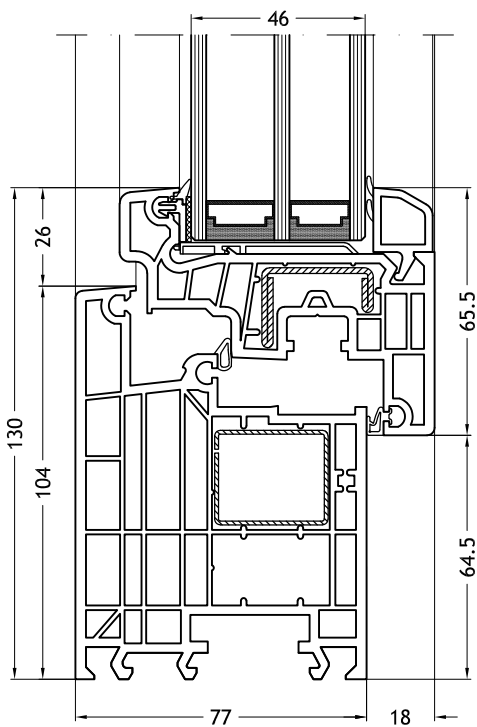
Telaio a L 963 con anta Slim-line
