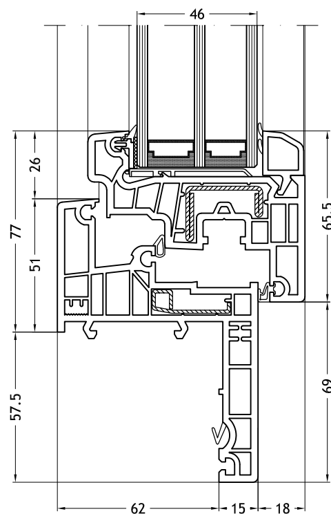
Telaio a Z 966 con anta Slim-line
