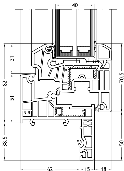
Telaio a Z 965 con anta Classic-line
