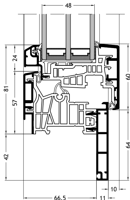
Soglia ribassata con anta Classic-line A27
