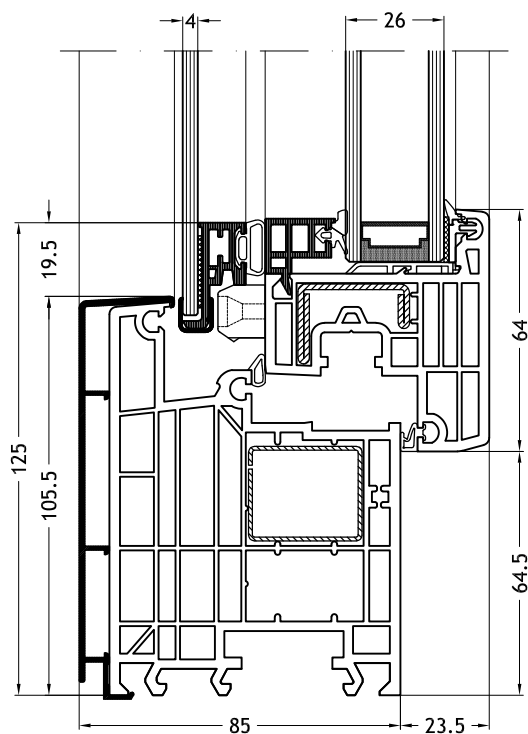
Telaio a L 963N con anta Nova-line Twin
