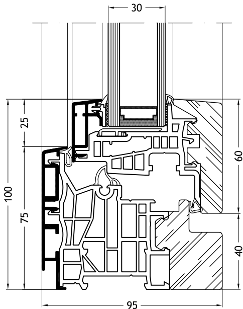
Telaio a L 9F1Z con anta Step-line
