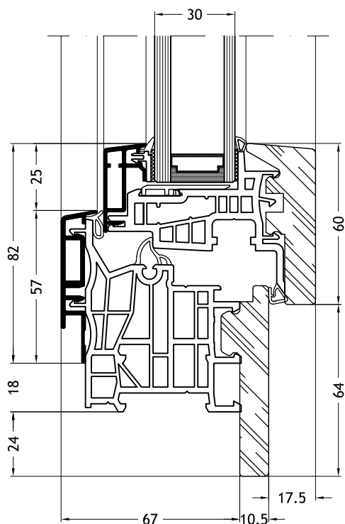
Telaio a L 9D1Y con anta Step-line
