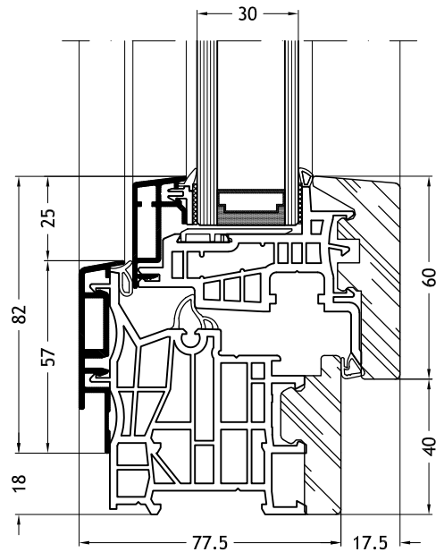
Telaio a L 9A1Y con anta Step-line
