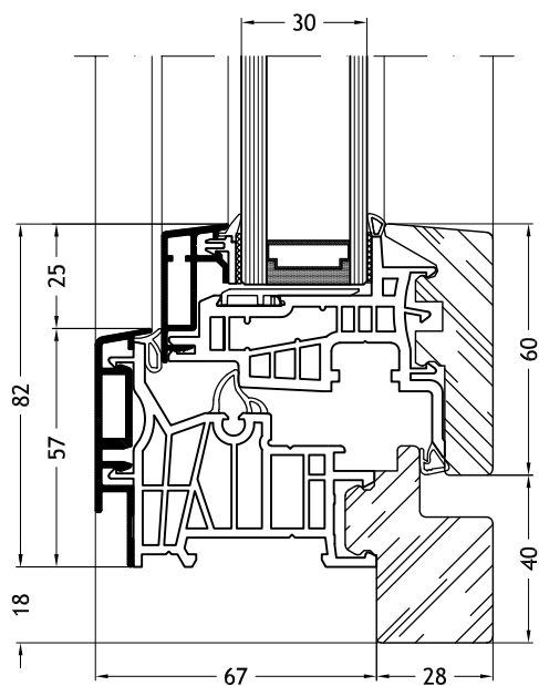
Telaio a Z 9F2Y con anta Step-line
