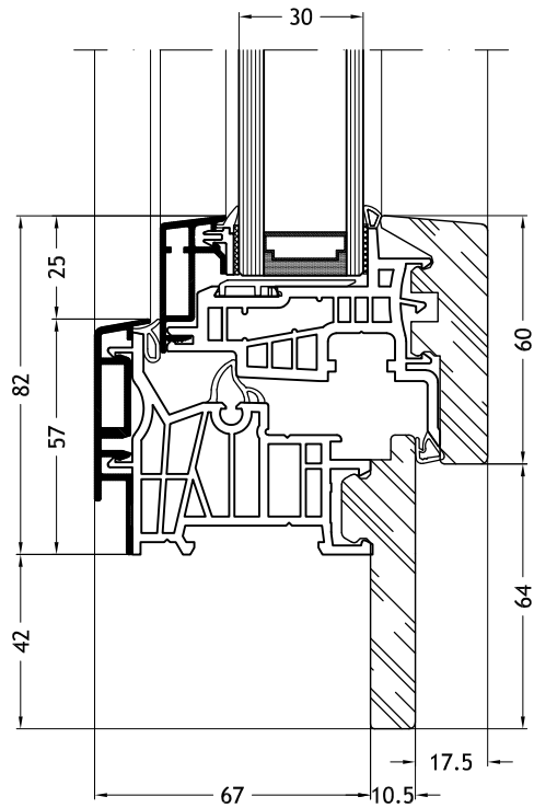
Telaio a Z 9D2Y con anta Step-line
