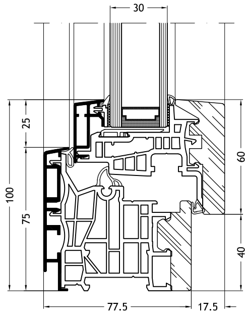
Telaio a L 9A1Z con anta Step-line
