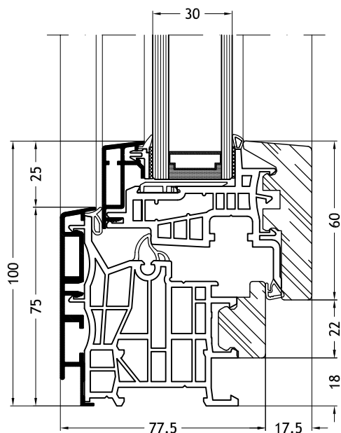
Telaio a L 9C1Z con anta Step-line
