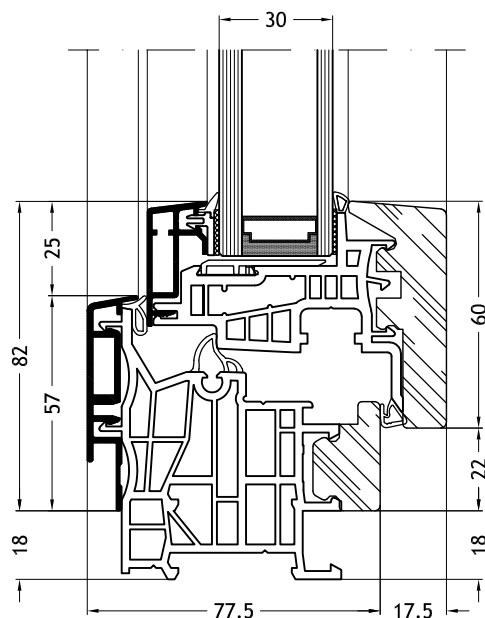
Telaio a L 9C1Y con anta Step-line
