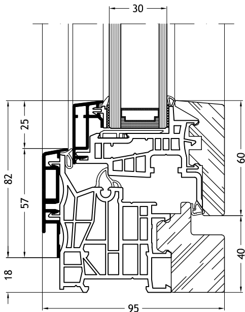
Telaio a L 9F1Y con anta Step-line
