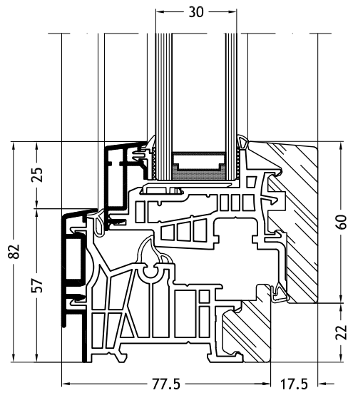
Telaio a Z 9C2Y con anta Step-line
