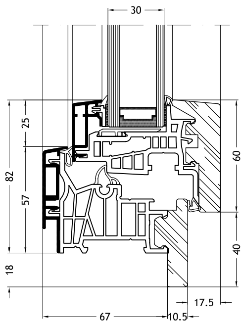
Telaio a Z 9A2Y con anta Step-line
