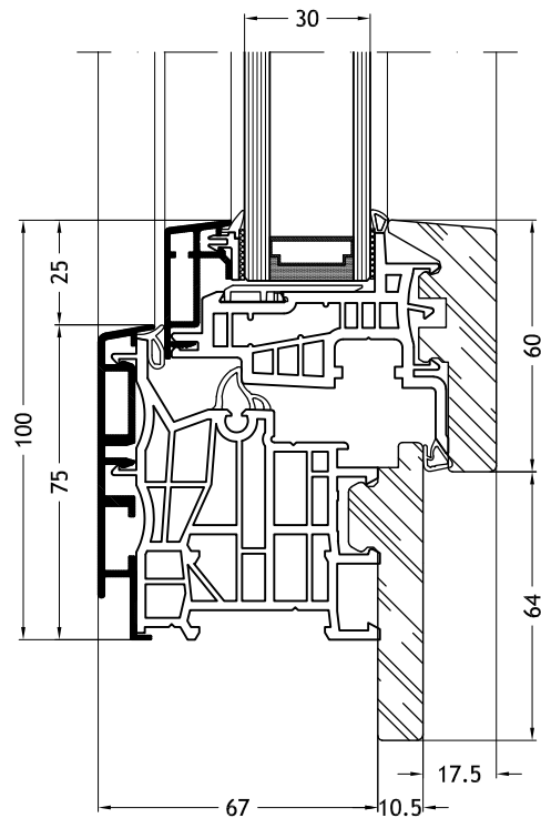
Telaio a L 9D1Z con anta Step-line
