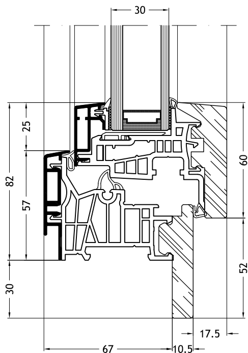
Telaio a Z 9B2Y con anta Step-line
