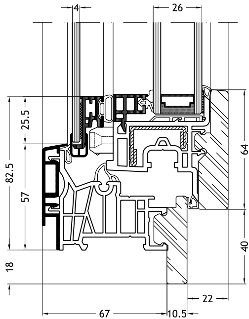
Telaio a Z 9A2Y con anta Nova-line Twin 9A32
