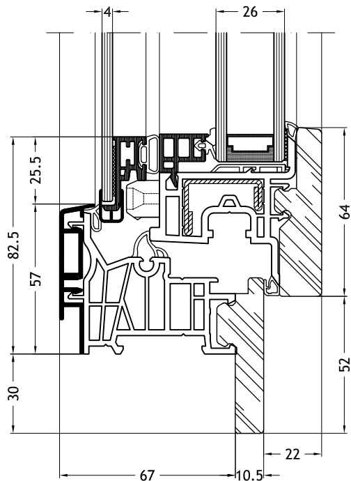
Telaio a Z 9B2Y con anta Nova-line Twin 9A32
