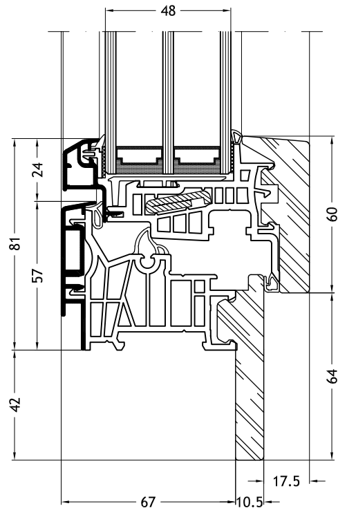
Telaio a Z 9D2Y con anta Classic-line 9A27
