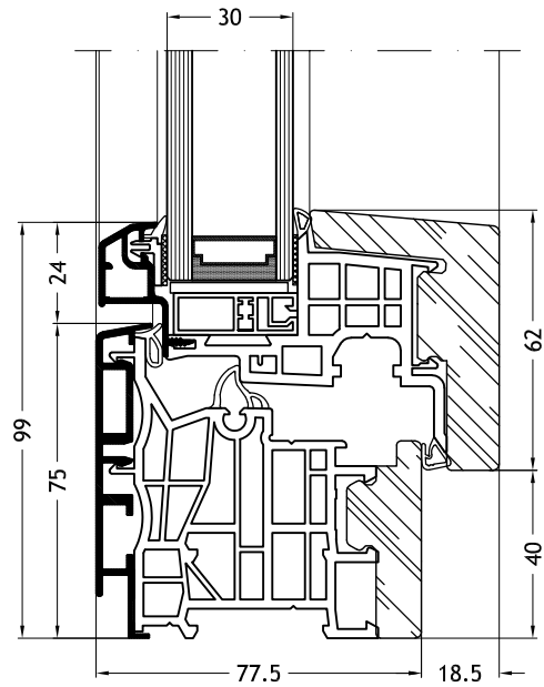
Telaio a L 9A1Z con anta Classic-line 9A26
