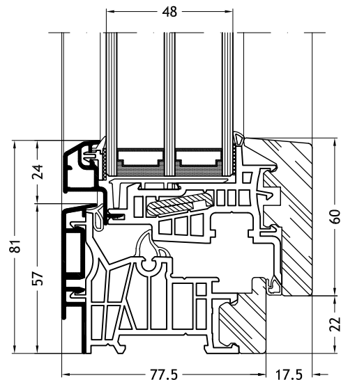
Telaio a Z 9C2Y con anta Classic-line 9A27
