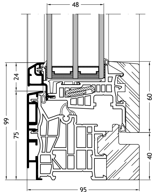
Telaio a L 9F1Z con anta Classic-line 9A27
