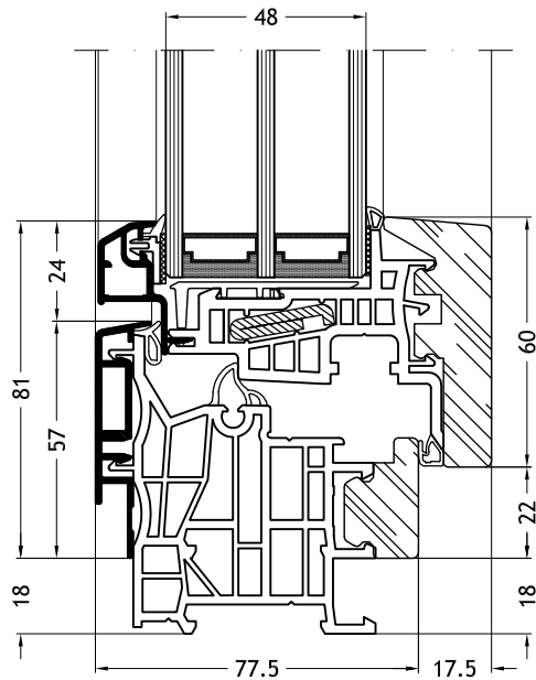
Telaio a L 9C1Y con anta Classic-line 9A27
