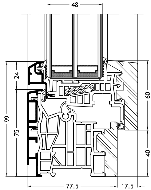
Telaio a L 9A1Z con anta Classic-line 9A27
