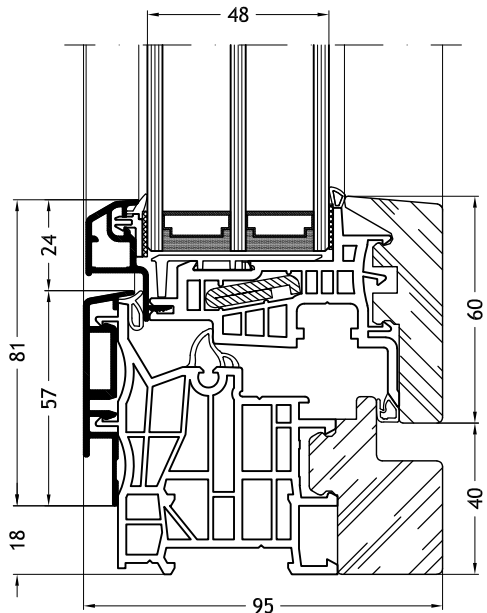
Telaio a Z 9F1Y con anta Classic-line 9A27
