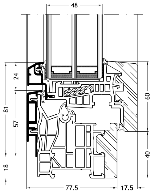
Telaio a L 9A1Y con anta Classic-line 9A27
