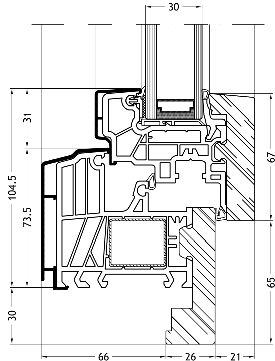
Telaio a Z 9D60K con anta Slim-line 9087K
