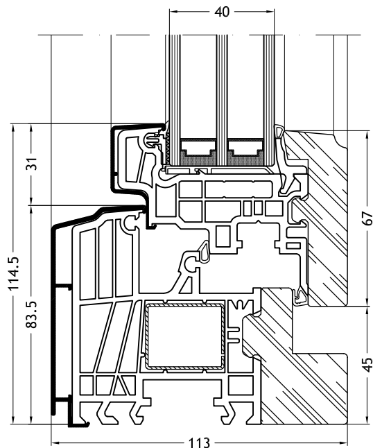
Telaio a L 9G43K con anta Slim-line 9S86K con rifinitura in stile
