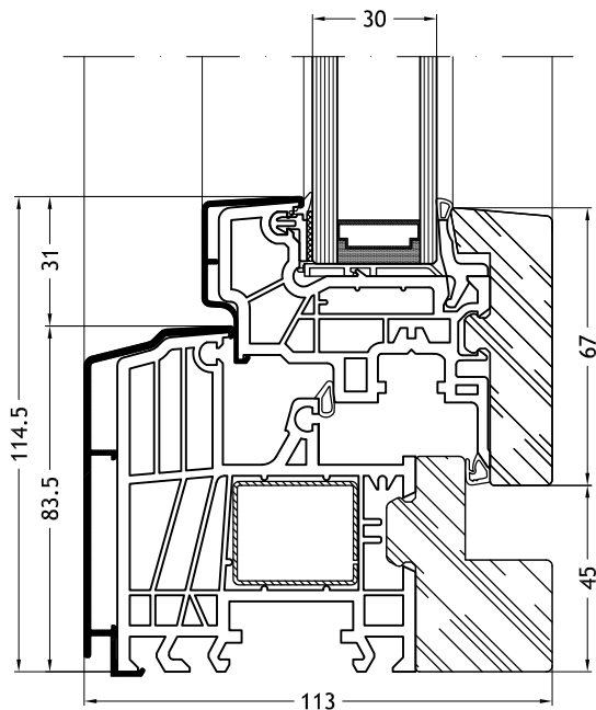
Telaio a L 9G43K con anta Slim-line 9087K
