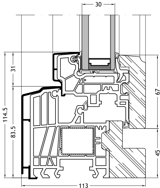
Telaio a L 9G43K con anta Slim-line 9S87K con rifinitura in stile
