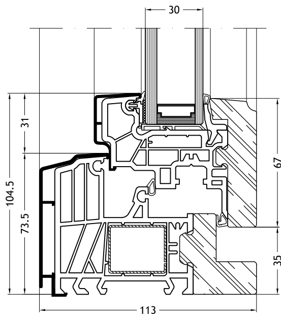
Telaio a L 9F60K con anta Slim-line 9S87K con rifinitura in stile
