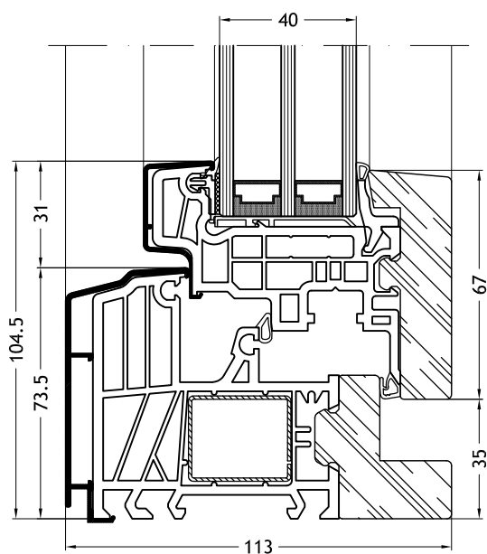
Telaio a L 9F60K con anta Slim-line 9086K
