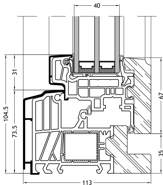
Telaio a L 9F60K con anta Slim-line 9S86K con rifinitura in stile
