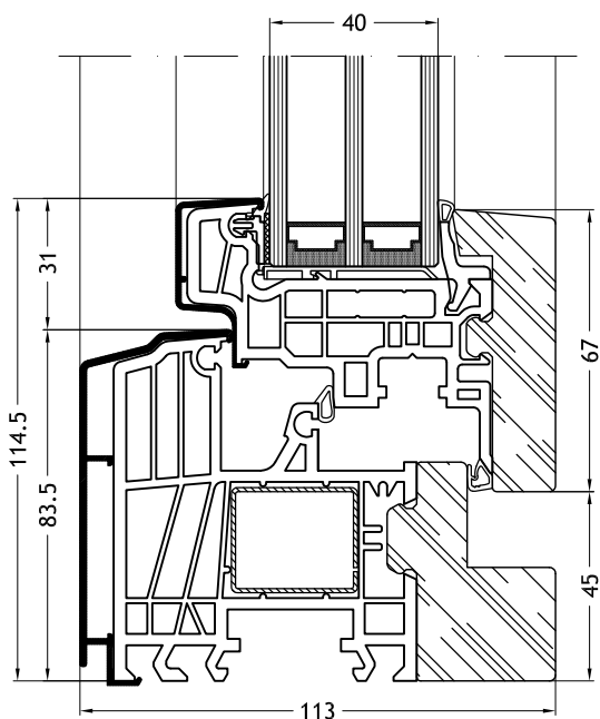
Telaio a L 9G43K con anta Slim-line 9086K
